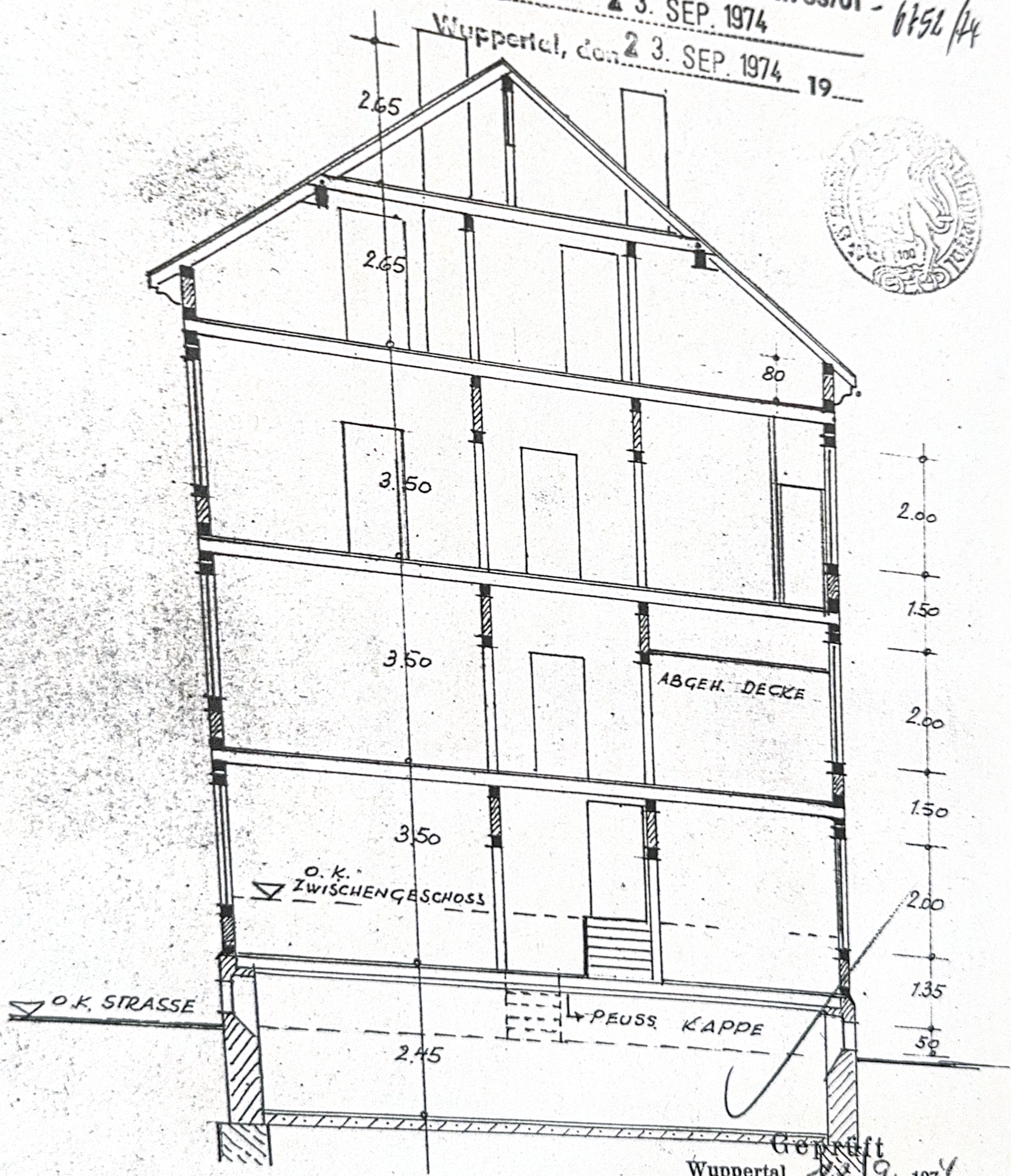
SCHNITT A - B
